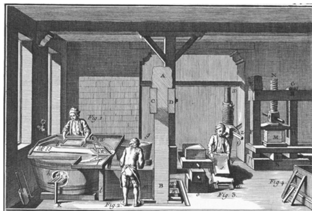
LA CUVE À OUVRER (Encyclopédie)
