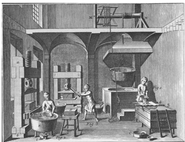
LA SALLE DE COLLAGE (Encyclopédie)
