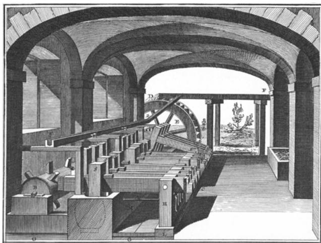
LA PILE À MAILLETS (Encyclopédie)
